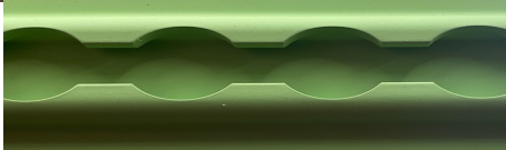
BAC1520-2193 7178-T6511 [DHCA] Chromic Acid Anodize per BAC 5019 CI 3 Primer BMS 10-11 Type I CI A Gr E per BAC 5736 Color: BAC 452 GREEN
